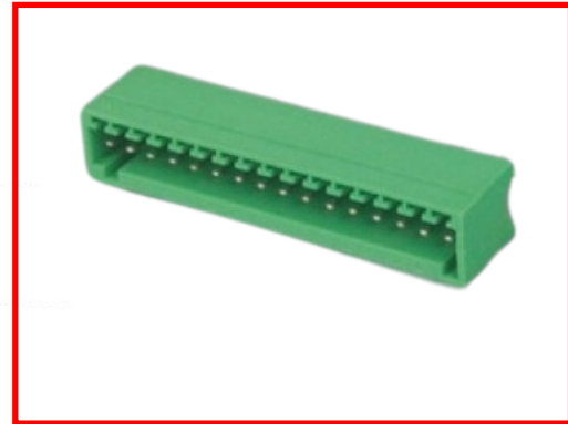
Borna macho acodada paso 2,50 mm circuito impreso
